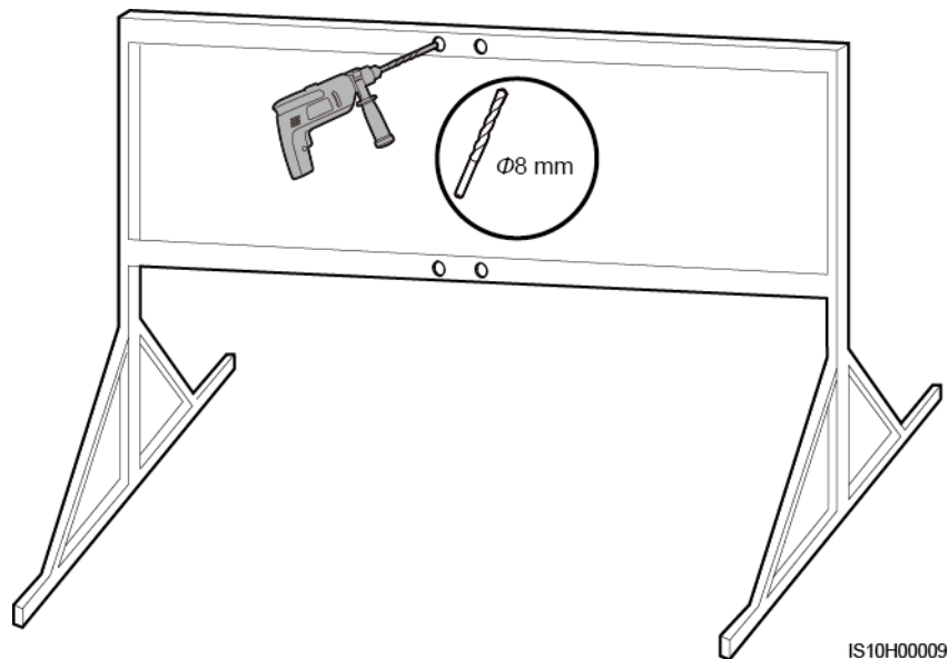
Figura 4-13 Foratura
