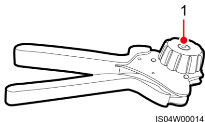
Figura 5-13 Crimpatrice (H4TC0003)
