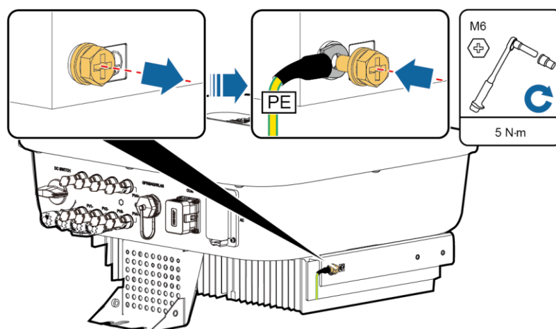
Figura 5-3 Collegamento del cavo PE
