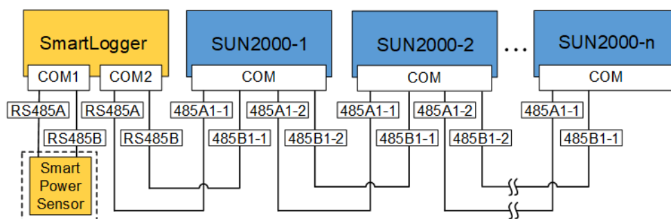
Figura 5-21 Rete SmartLogger1000A
