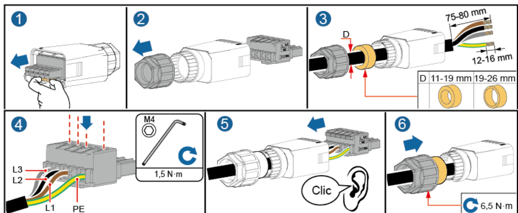
Figura 5-7 Cavo a quattro anime (L1, L2, L3 e PE)
