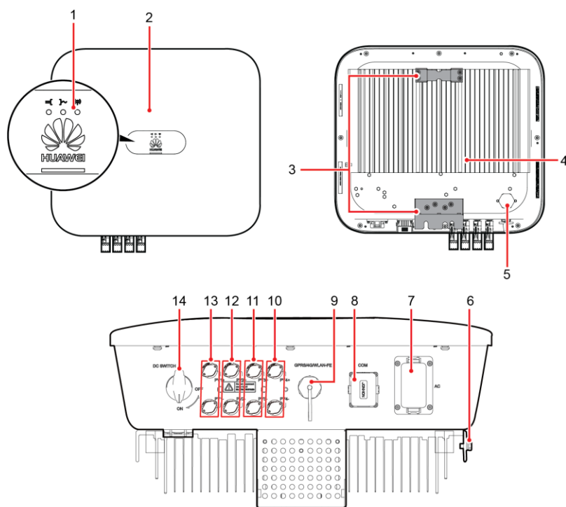
Figura 2-5 Aspetto
