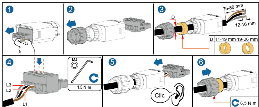
Figura 5-6 Cavo a tre anime (L1, L2 e L3)
