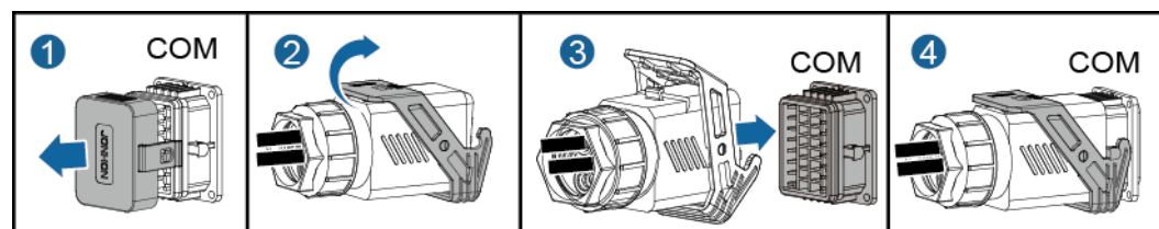
Figura 5-23 Fissaggio del connettore del cavo di segnale
