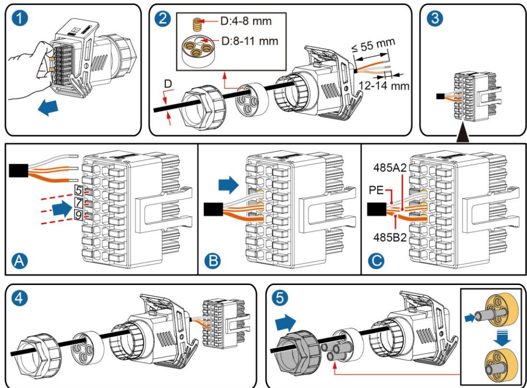
Figura 5-26 Installazione del cavo
