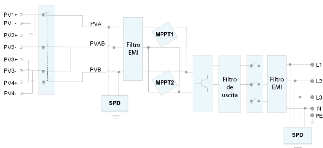
Figura 2-7 Schema concettuale del SUN2000
