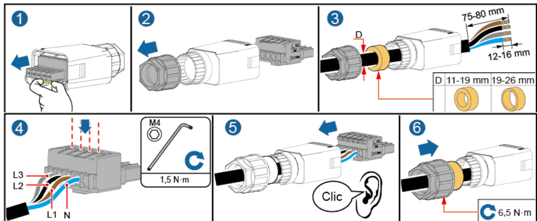
Figura 5-8 Cavo a quattro anime (L1, L2, L3 e N)
