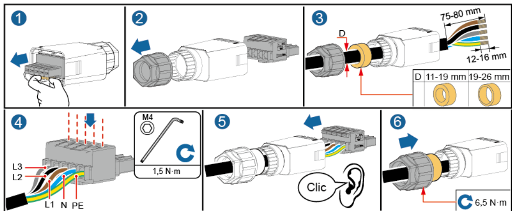
Figura 5-9 Cavo a cinque anime (L1, L2, L3, N e PE)
