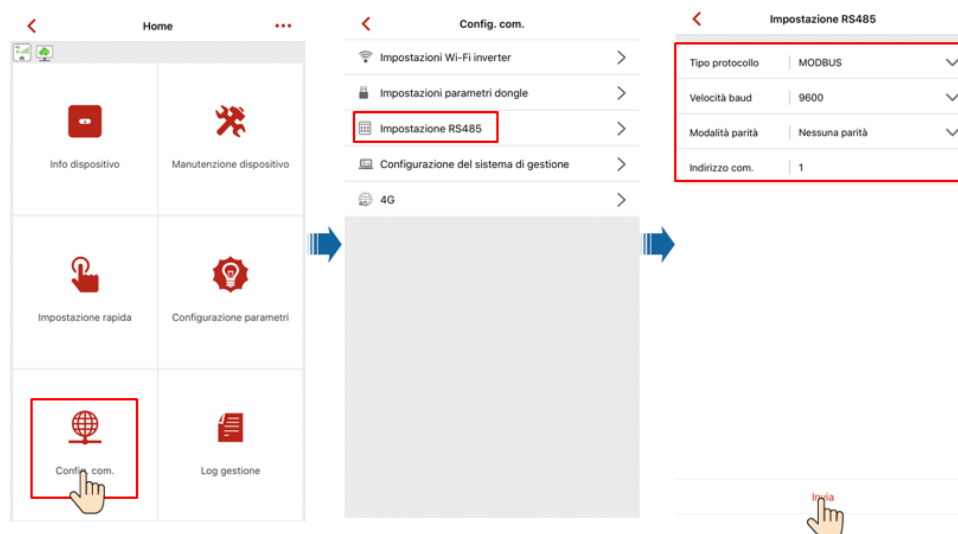
Figura 6-9 Impostazione RS485
