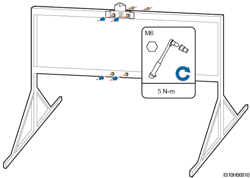
Figura 4-14 Fissare la staffa di montaggio
