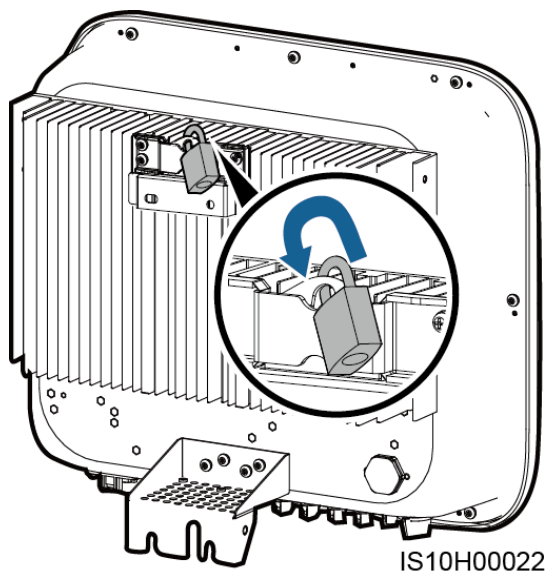
Figura 4-11 Installazione del lucchetto
