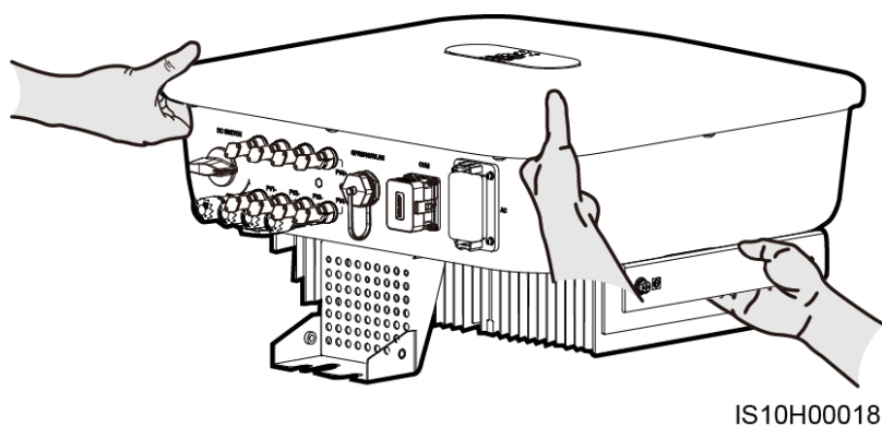
Figura 4-6 Spostamento di un inverter
