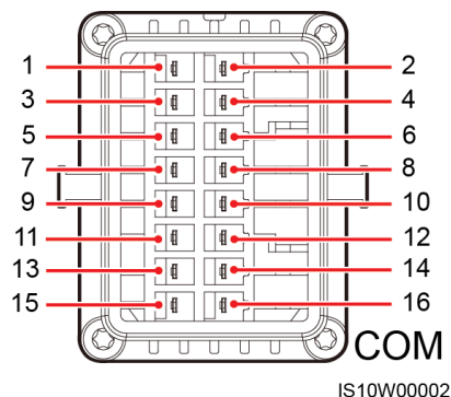
Figura 5-19 Definizioni di segnale
