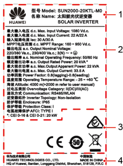
Figura 2-6 Targhetta (SUN2000-20KTL-M0 come esempio)
