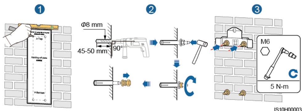
Figura 4-9 Installazione della staffa di montaggio
