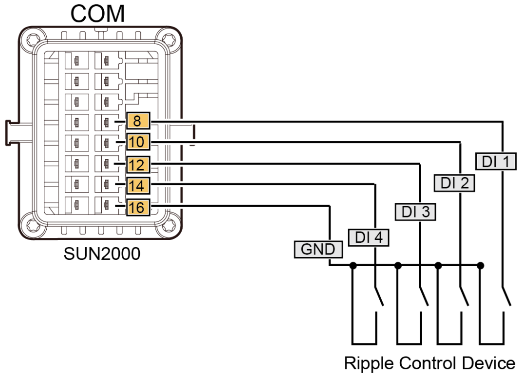
Figura 5-28 Collegamento dei cavi
