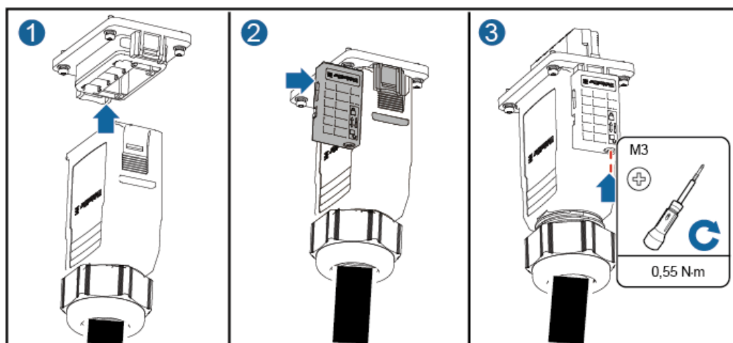
Figura 5-10 Fissaggio del connettore CA
