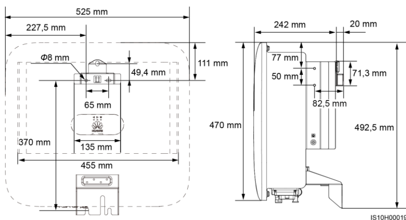
Figura 4-7 Dimensioni della staffa di montaggio
