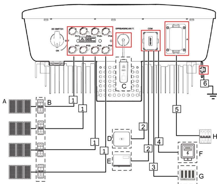
Figura 5-1 Collegamenti via cavo del SUN2000 (opzionale nei riquadri tratteggiati)
