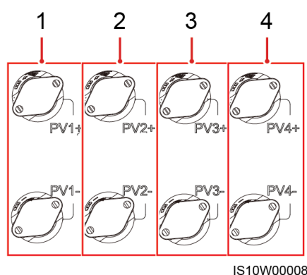
Figura 5-12 Terminali
