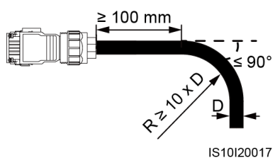
Figura 5-11 Instradamento dei cavi
