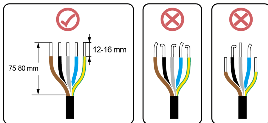
Figura 5-5 Requisiti di spelatura
