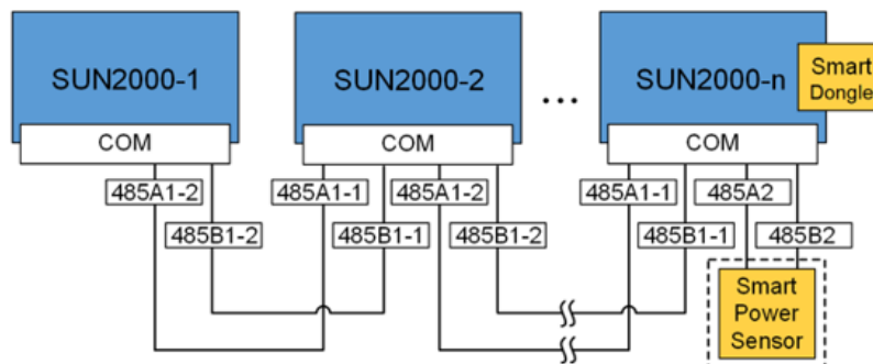
Figura 5-20 Rete SmartDongle
