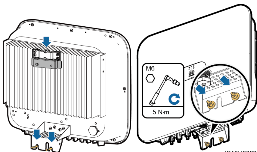
Figura 4-10 Installazione del SUN2000
