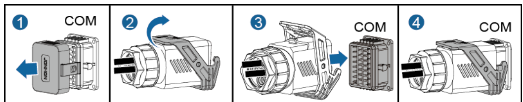
Figura 5-27 Fissaggio del connettore del cavo di segnale
