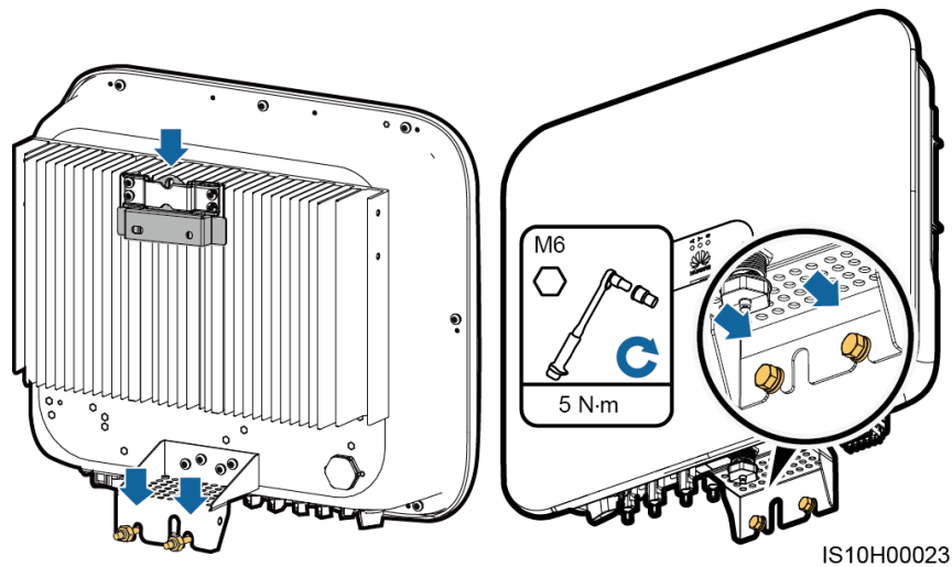
Figura 4-15 Installazione del SUN2000
