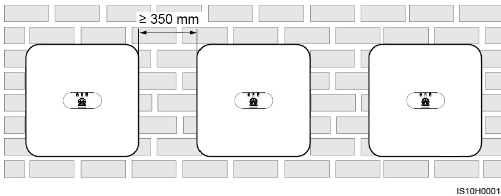
Figura 4-3 Installazione in posizione orizzontale (consigliata)
