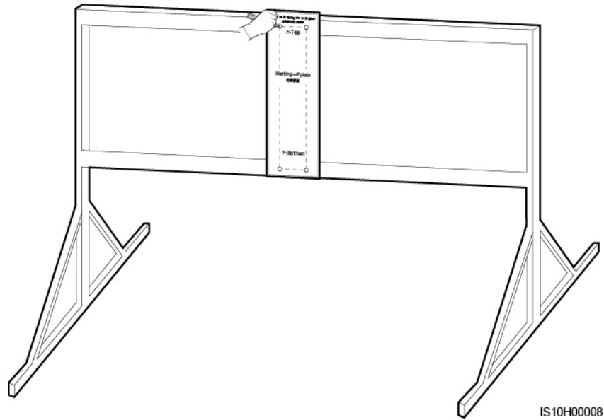
Figura 4-12 Determinazione della posizione dei fori
