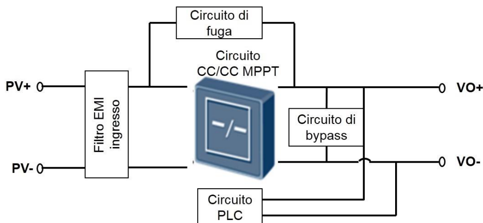
Figura 2-2 Diagramma concettuale
