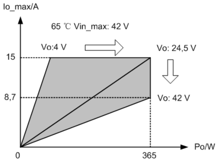
Figura A-3 Curva di relazione I_{o\_max} - P_o ( 65^\circ\text{C} , V_{in\_max} = 42\text{ V} )
