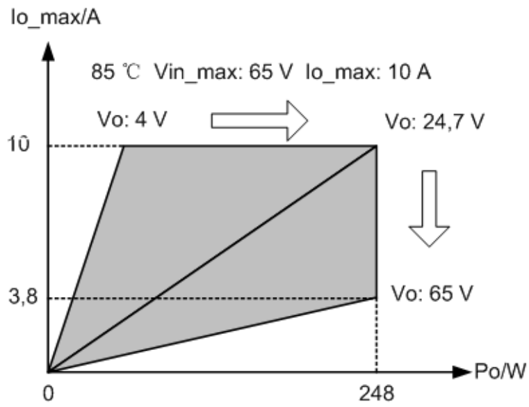
Figura A-5 Curva di relazione I_{o\_max} - P_o ( 85^\circ\text{C} , V_{in\_max} = 65\text{ V} , I_{o\_max} = 10\text{ A} )
