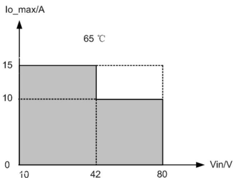
Figura A-2 Curva di relazione I_{o\_max} - V_{in} (65°C)
