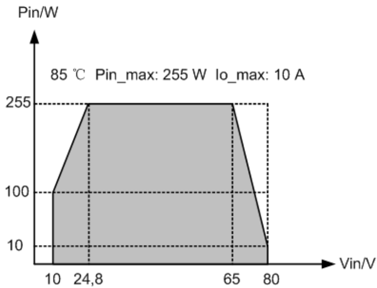
Figura A-6 Curva di relazione P_{in} - V_{in} ( 85^\circ\text{C} , P_{in\_max} = 255\text{ W} , I_{o\_max} = 10\text{ A} )
