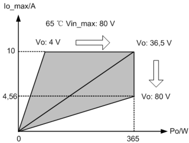
Figura A-4 Curva di relazione I_{o\_max} - P_o ( 65^\circ\text{C} , V_{in\_max} = 80\text{ V} )
