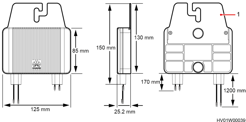
Figura 2-7 Dimensioni del prodotto
